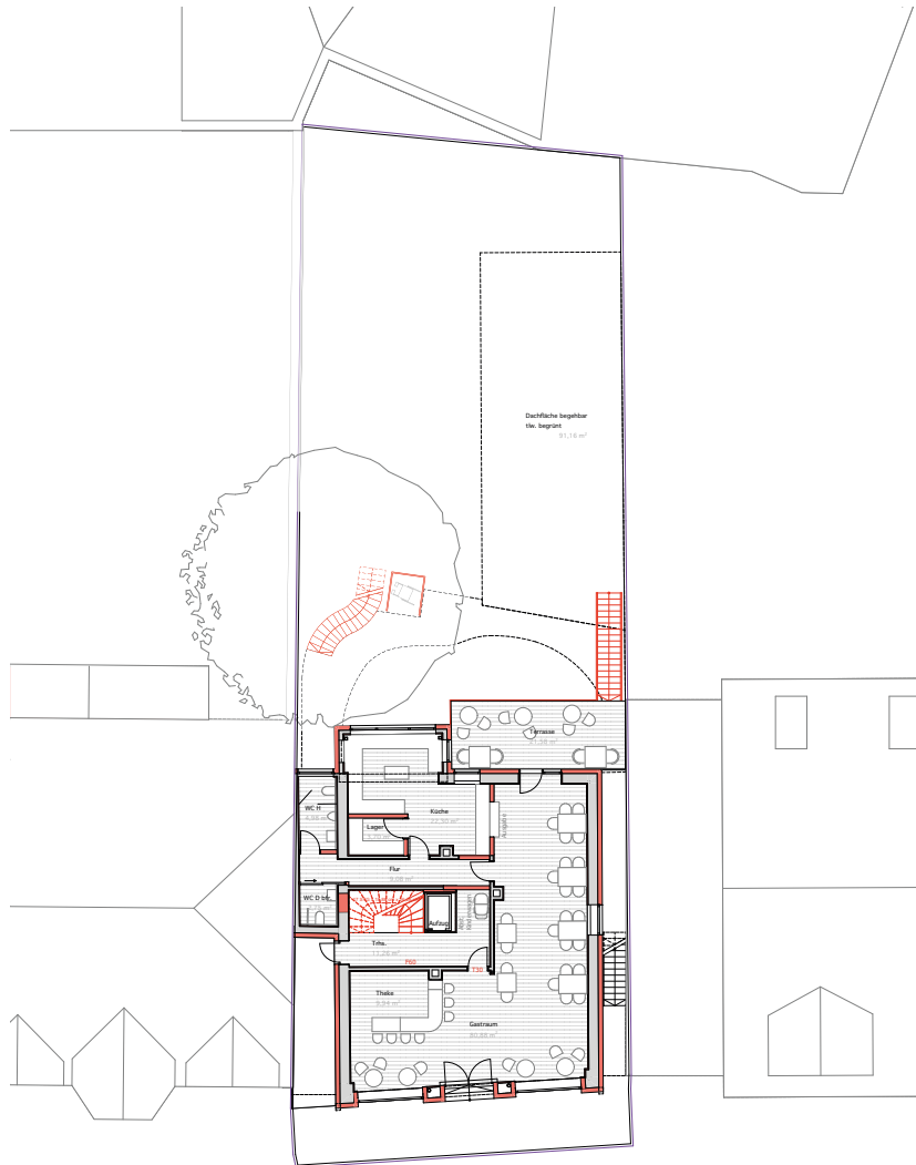
grundriss / eg
