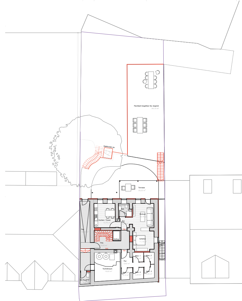
grundriss / ug
